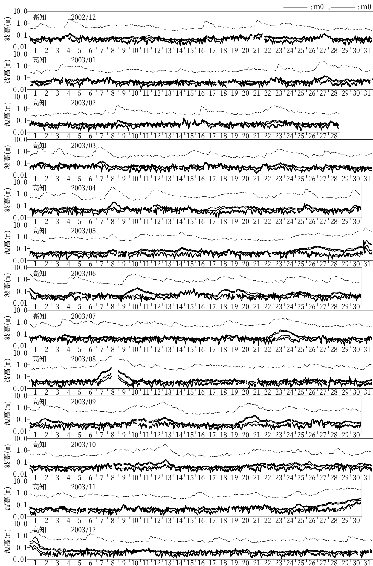
図-10.46 長周期波高の経時変化図（高知）
