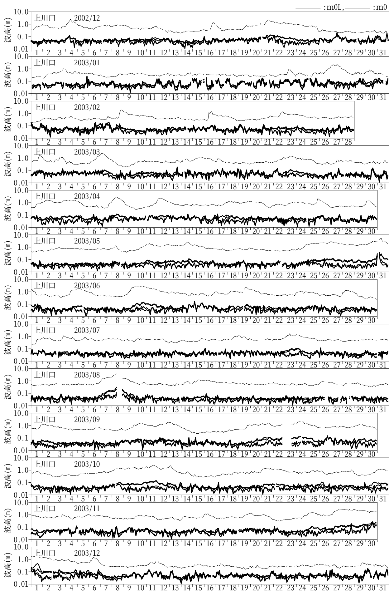
図-10.47 長周期波高の経時変化図（上川口）
