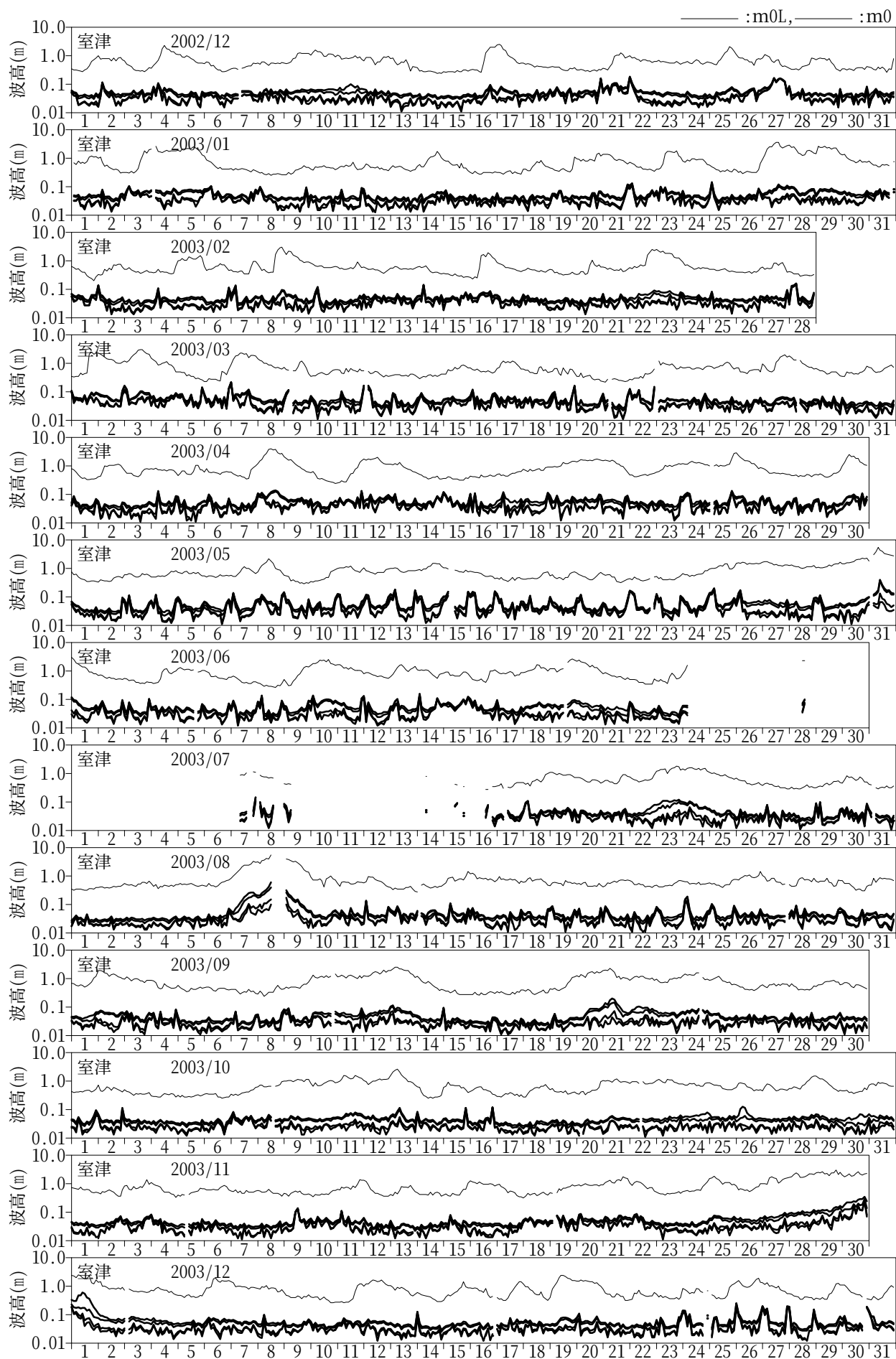
図-10.45 長周期波高の経時変化図（室津）
