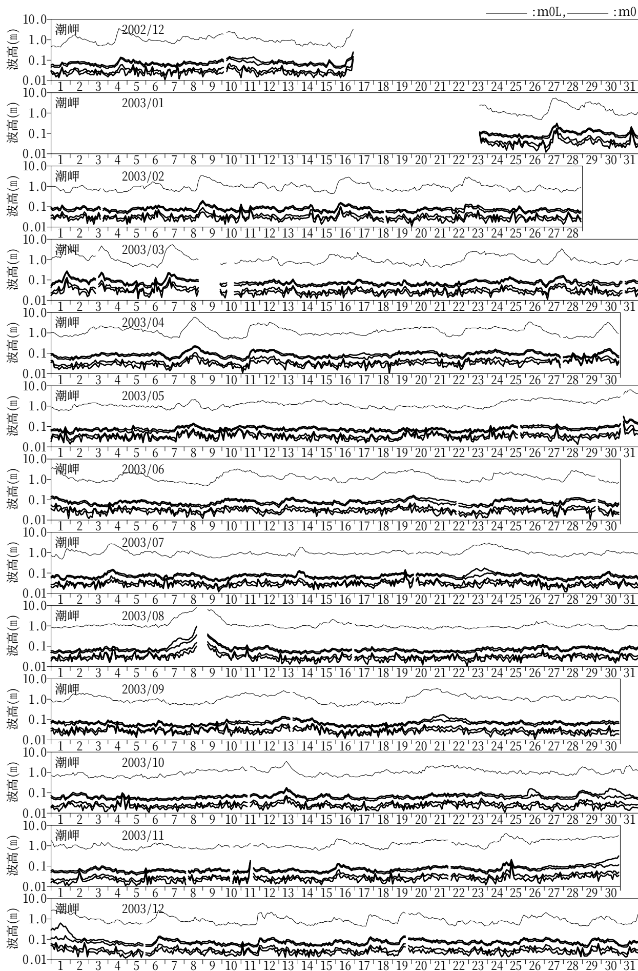
図-10.42 長周期波高の経時変化図（潮岬）
