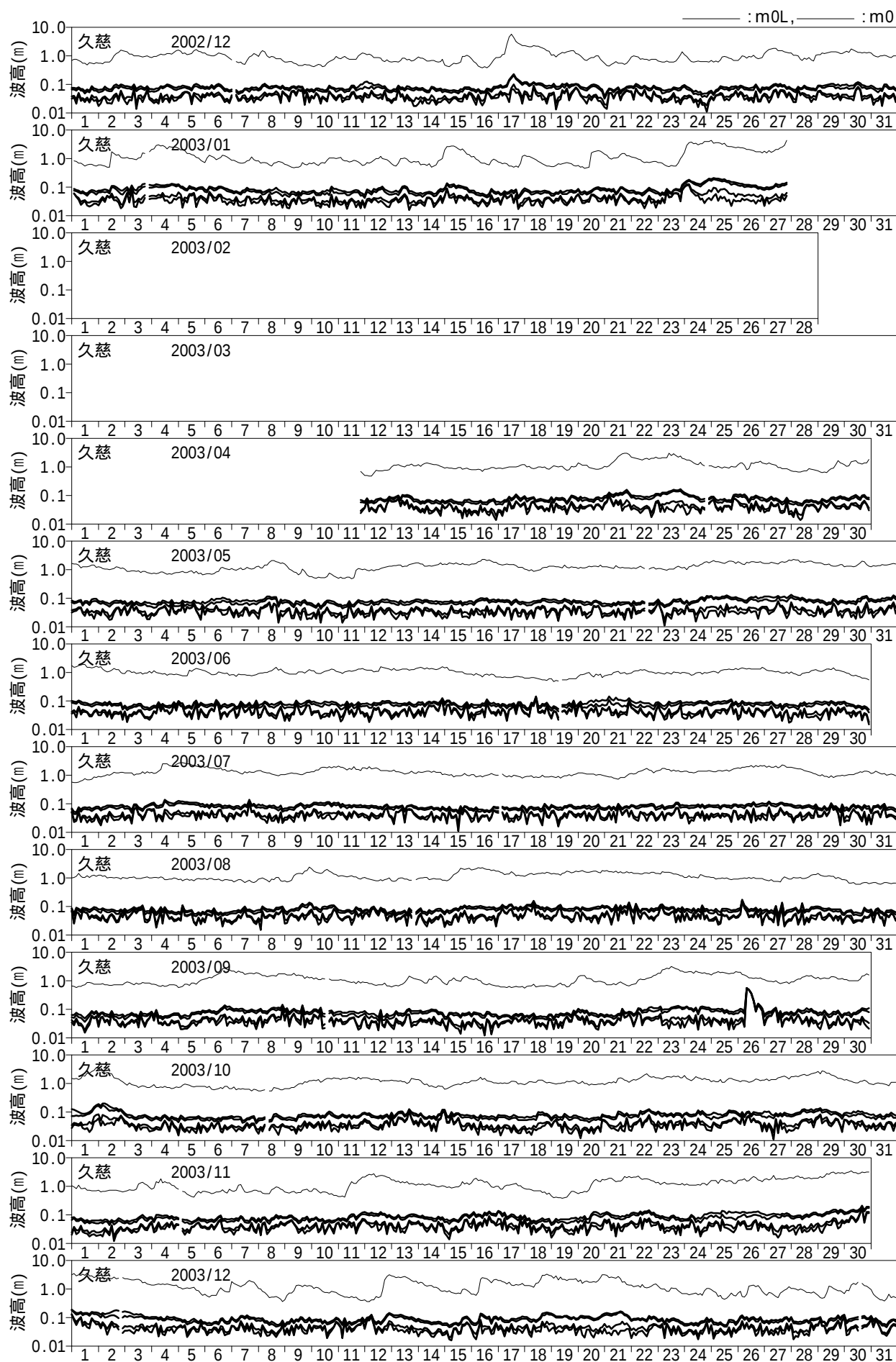
図 - 10.27 長周期波高の経時変化図 (久慈)
