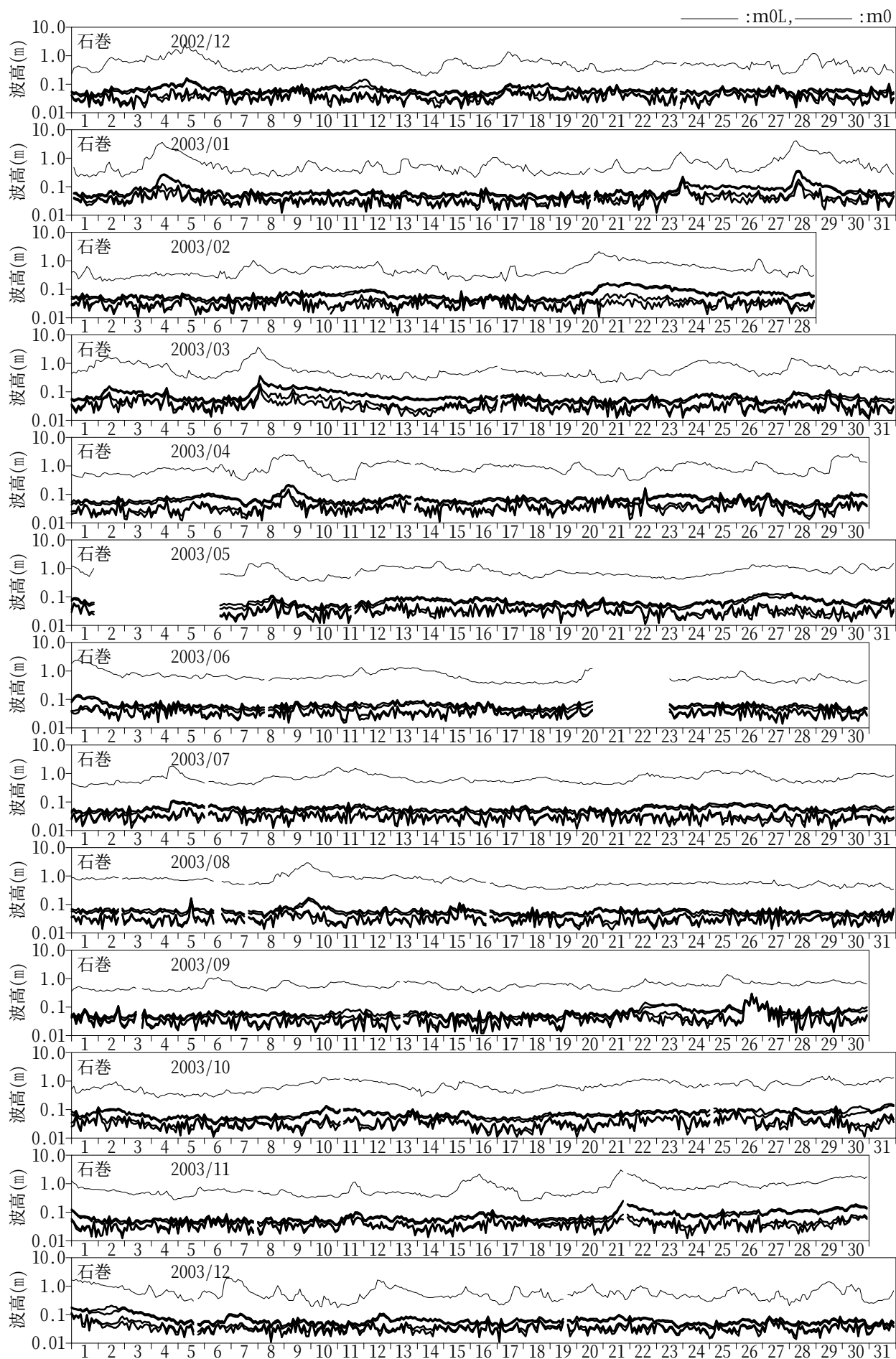
図-10.29 長周期波高の経時変化図 (石巻)
