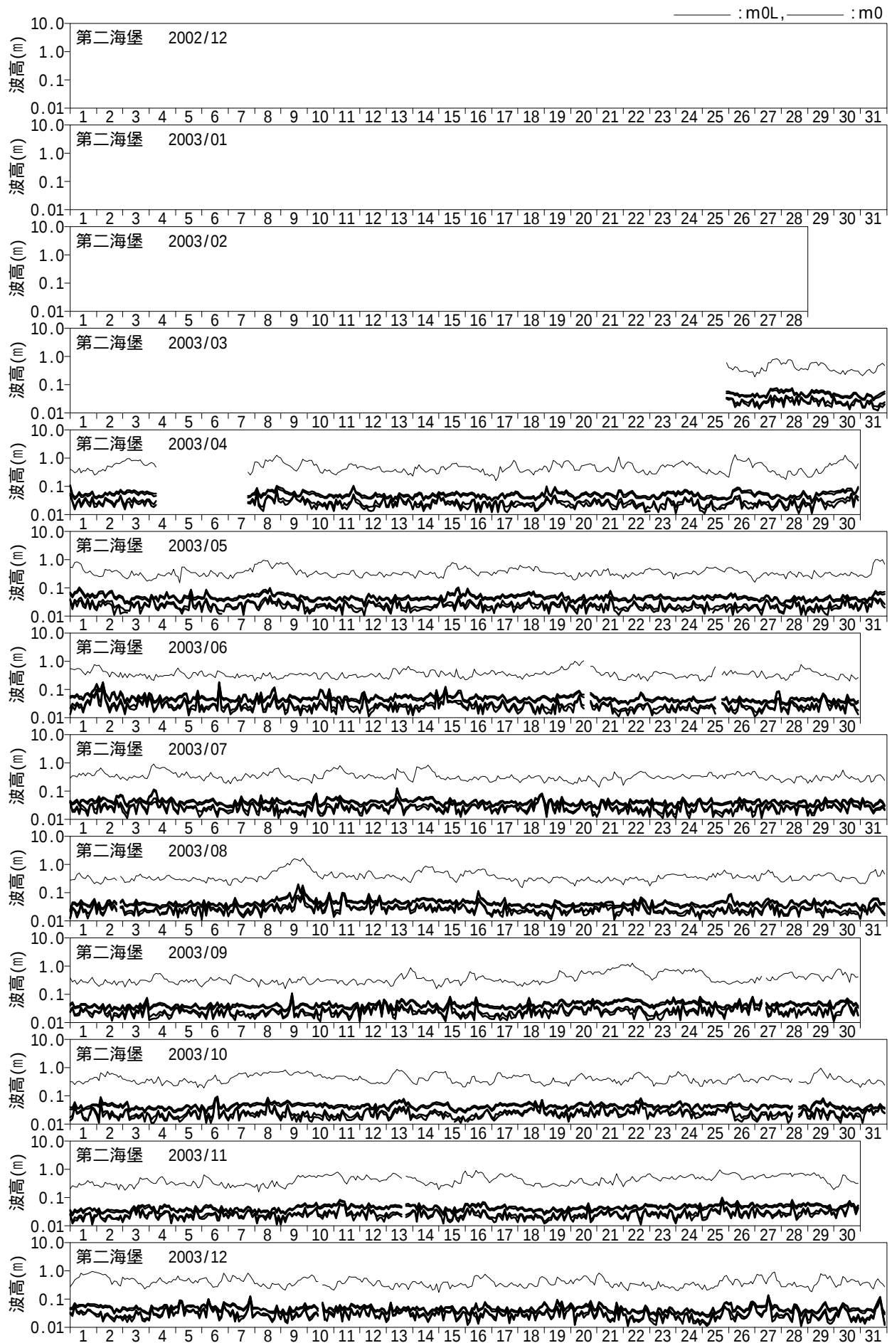
図 - 10.35 長周期波高の経時変化図 (第二海堡)
