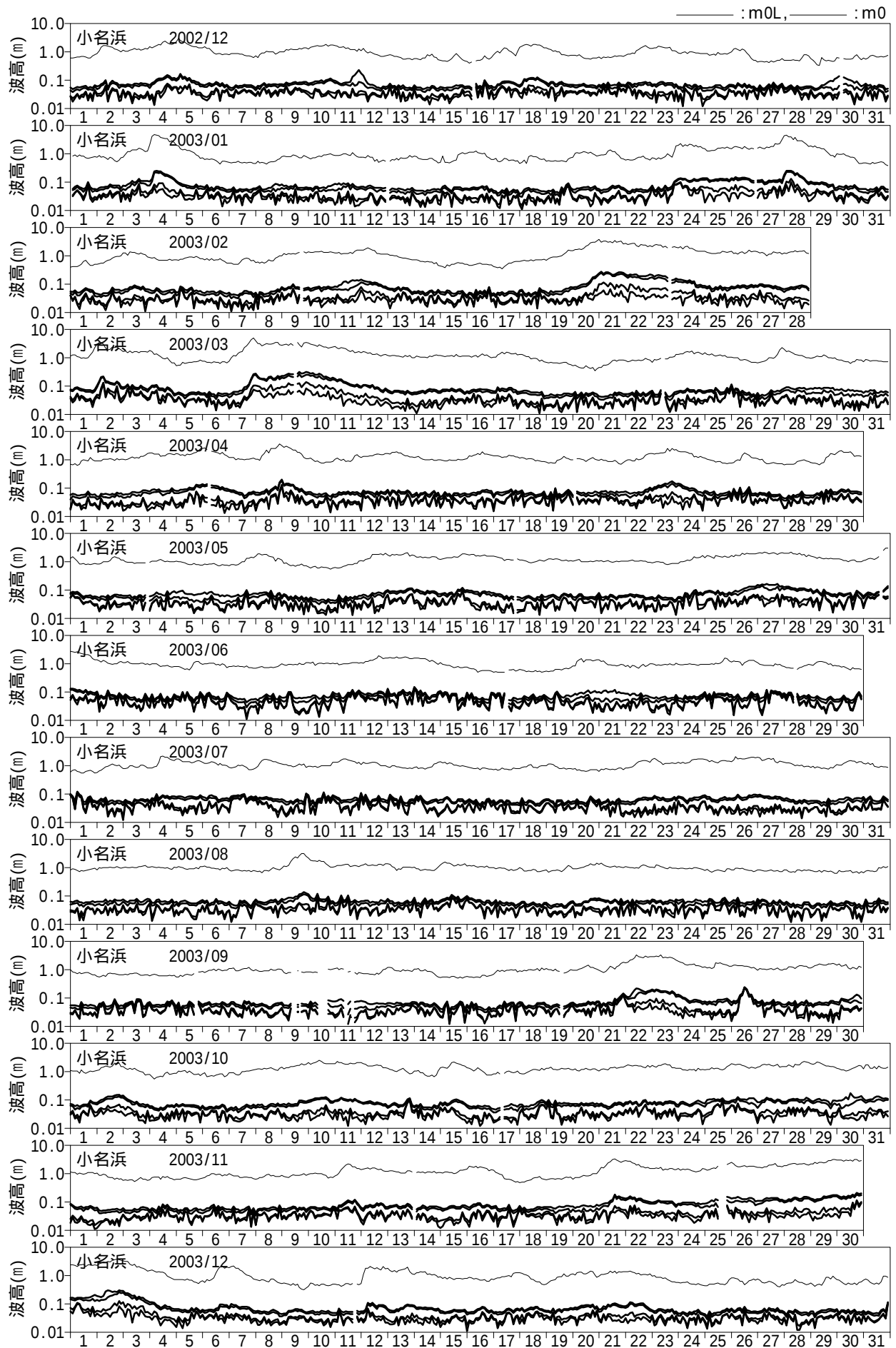
図 - 10.32 長周期波高の経時変化図 (小名浜)
