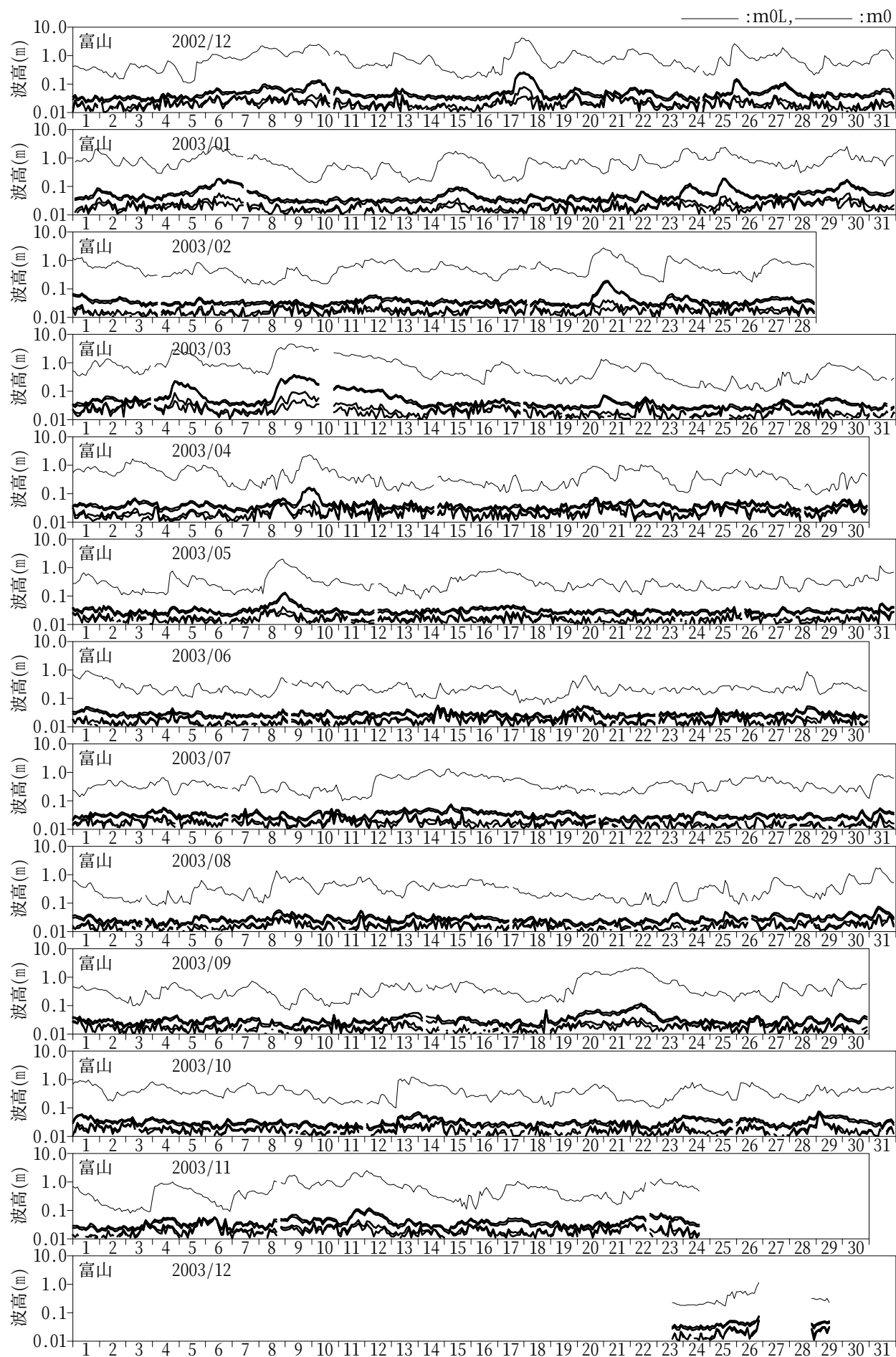
図-10.8 長周期波高の経時変化図（富山）
