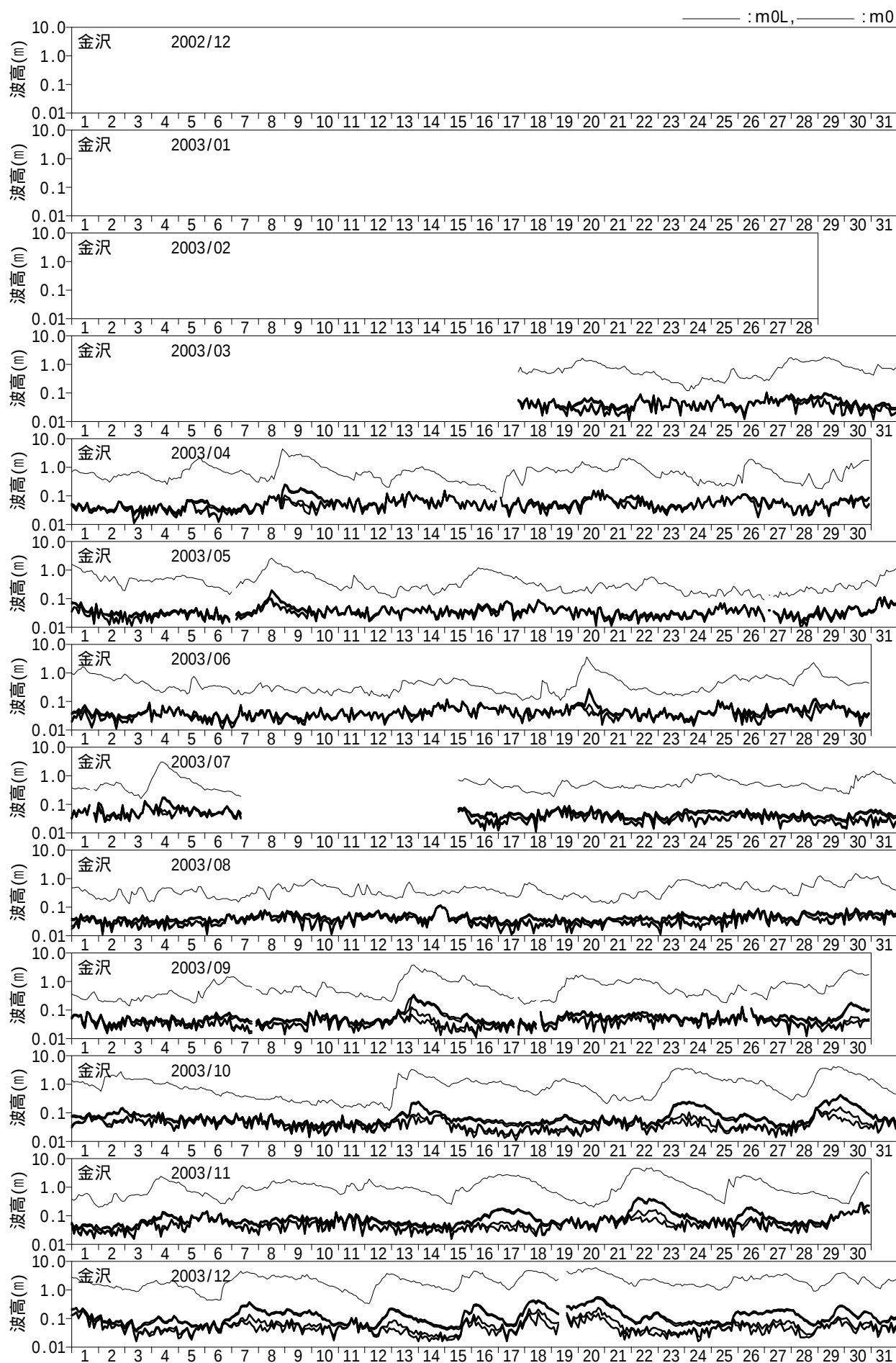
図 - 10.11 長周期波高の経時変化図（金沢）
