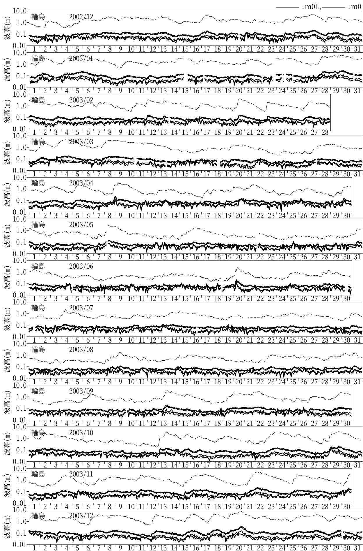
図-10.10 長周期波高の経時変化図（輪島）
