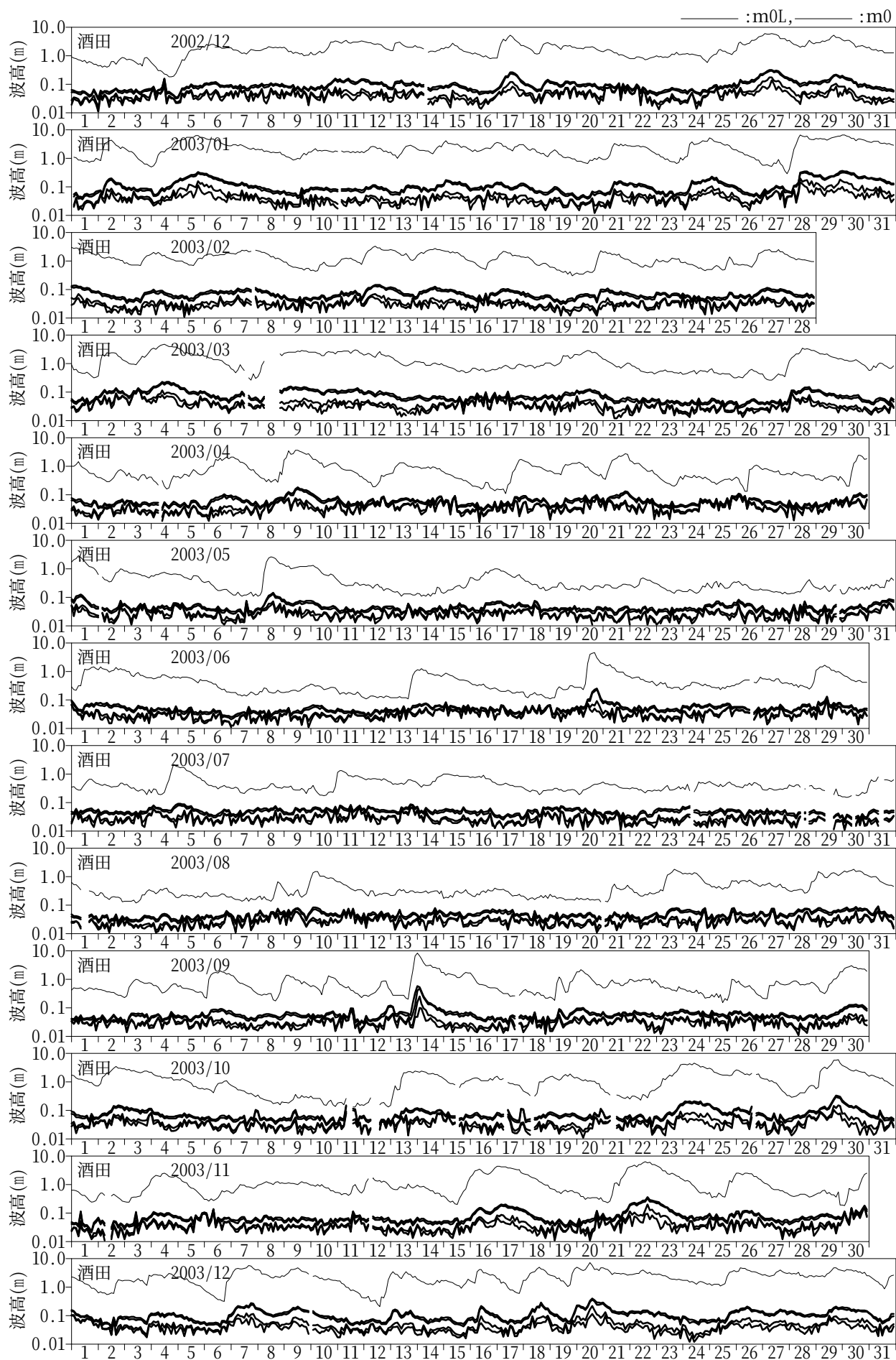
図-10.5 長周期波高の経時変化図（酒田）
