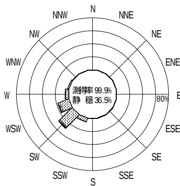
図 - 8.19 伊王島 波高・波向別出現頻度図
