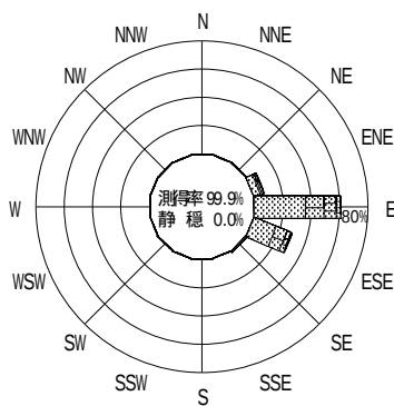
図 - 8.25 むつ小川原 波高・波向別出現頻度図
