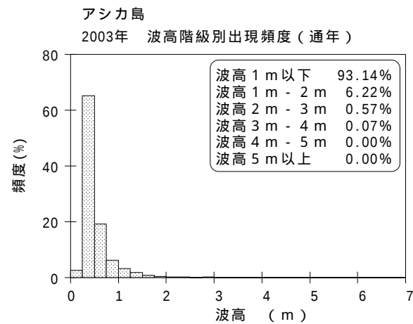
図 - 7.36 アシカ島 波候特性図
