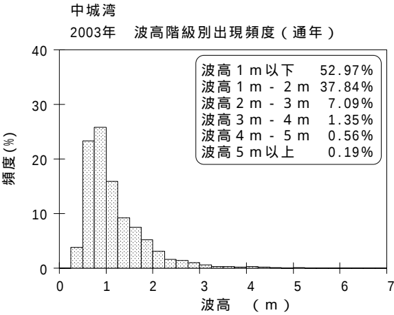
図 - 7.53 中城湾 波候特性図
