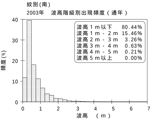
図 - 7.22 紋別(南) 波候特性図
