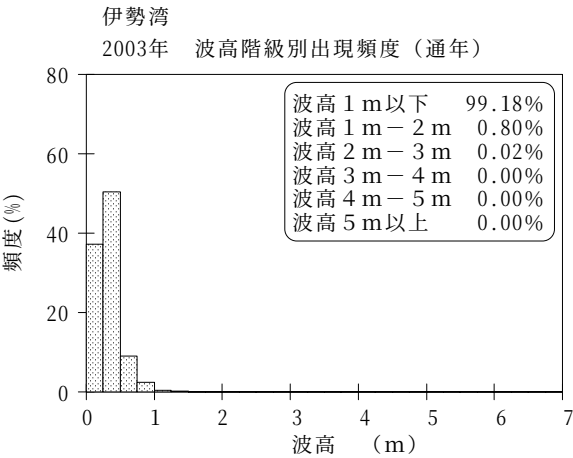
図-7.41 伊勢湾 波候特性図
