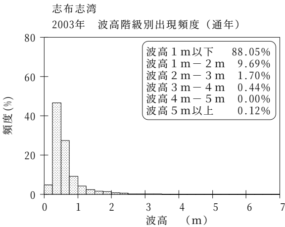
図-7.51 志布志湾 波候特性図
