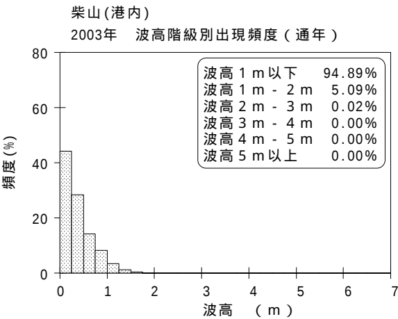
図 - 7.13 柴山(港内) 波候特性図
