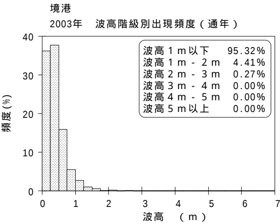
図 - 7.15 境港 波候特性図
