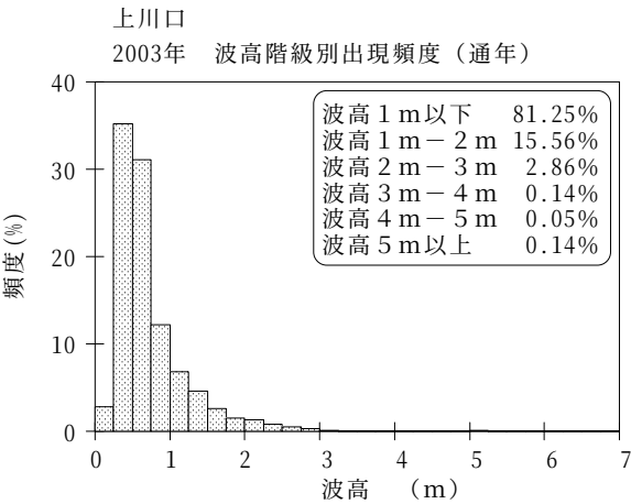
図-7.47 上川口 波候特性図
