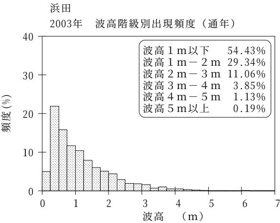
図-7.16 浜田 波候特性図
