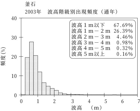
図-7.28 釜石 波候特性図
