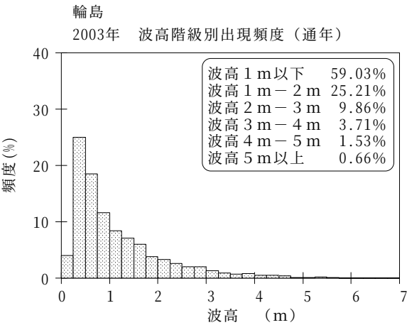
図-7.10 輪島 波候特性図
