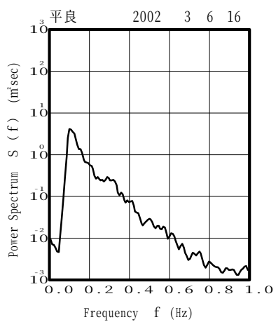
付図-B.3.54 平良 代表的な高波期間中のスペクトル
