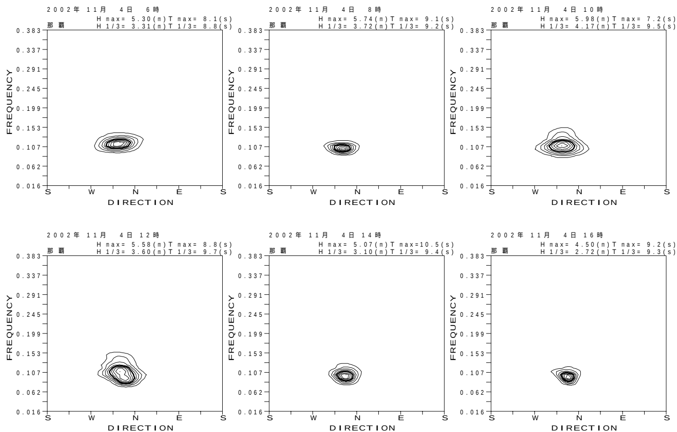
付図 - B.3.21 那覇 代表的な高波期間中の方向スペクトル
