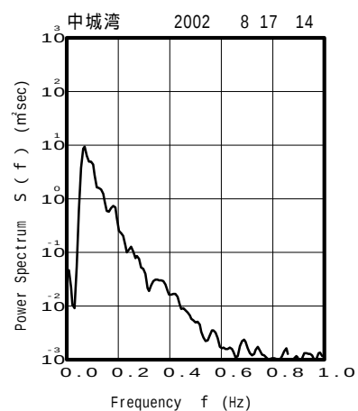
付図 - B.3.53 中城湾 代表的な高波期間中のスペクトル
