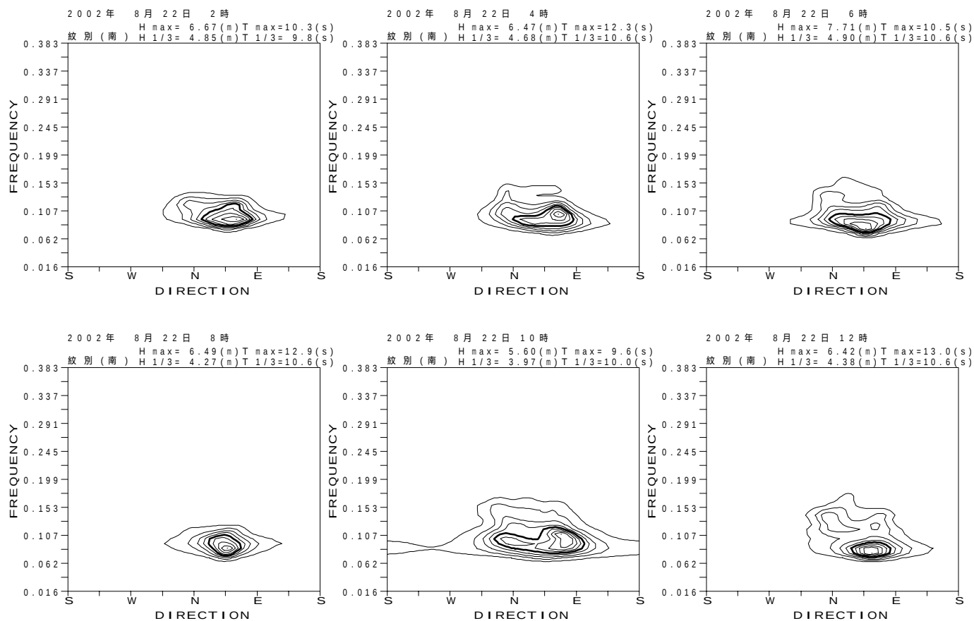
付図 - B.3.22 紋別(南) 代表的な高波期間中の方向スペクトル
