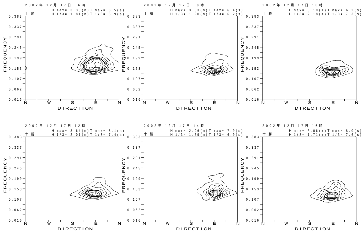
付図 - B.3.23 十勝 代表的な高波期間中の方向スペクトル
