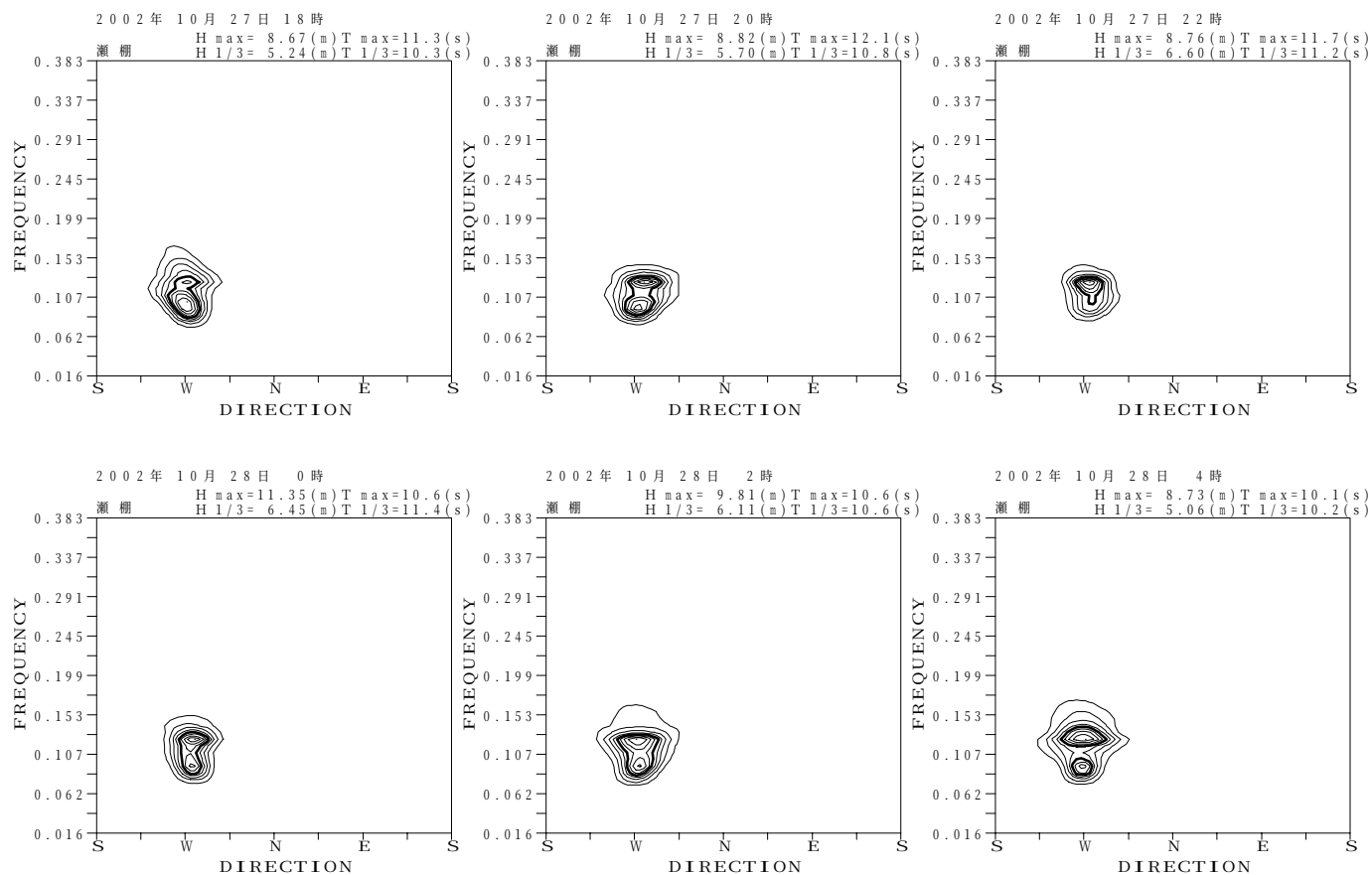
付図－B.3.2 瀬棚 代表的な高波期間中の方向スペクトル
