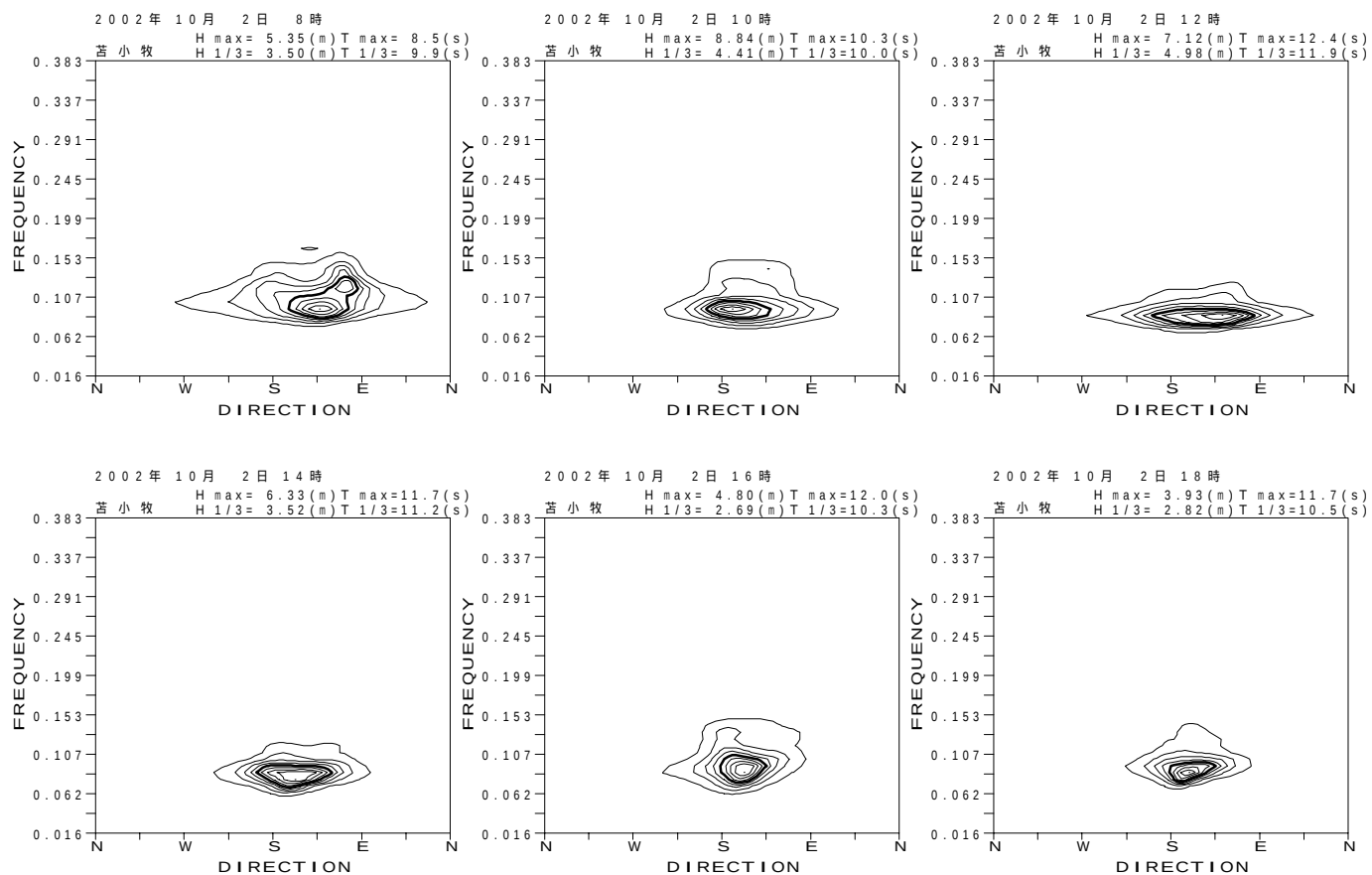
付図 - B.3.24 苦小牧 代表的な高波期間中の方向スペクトル
