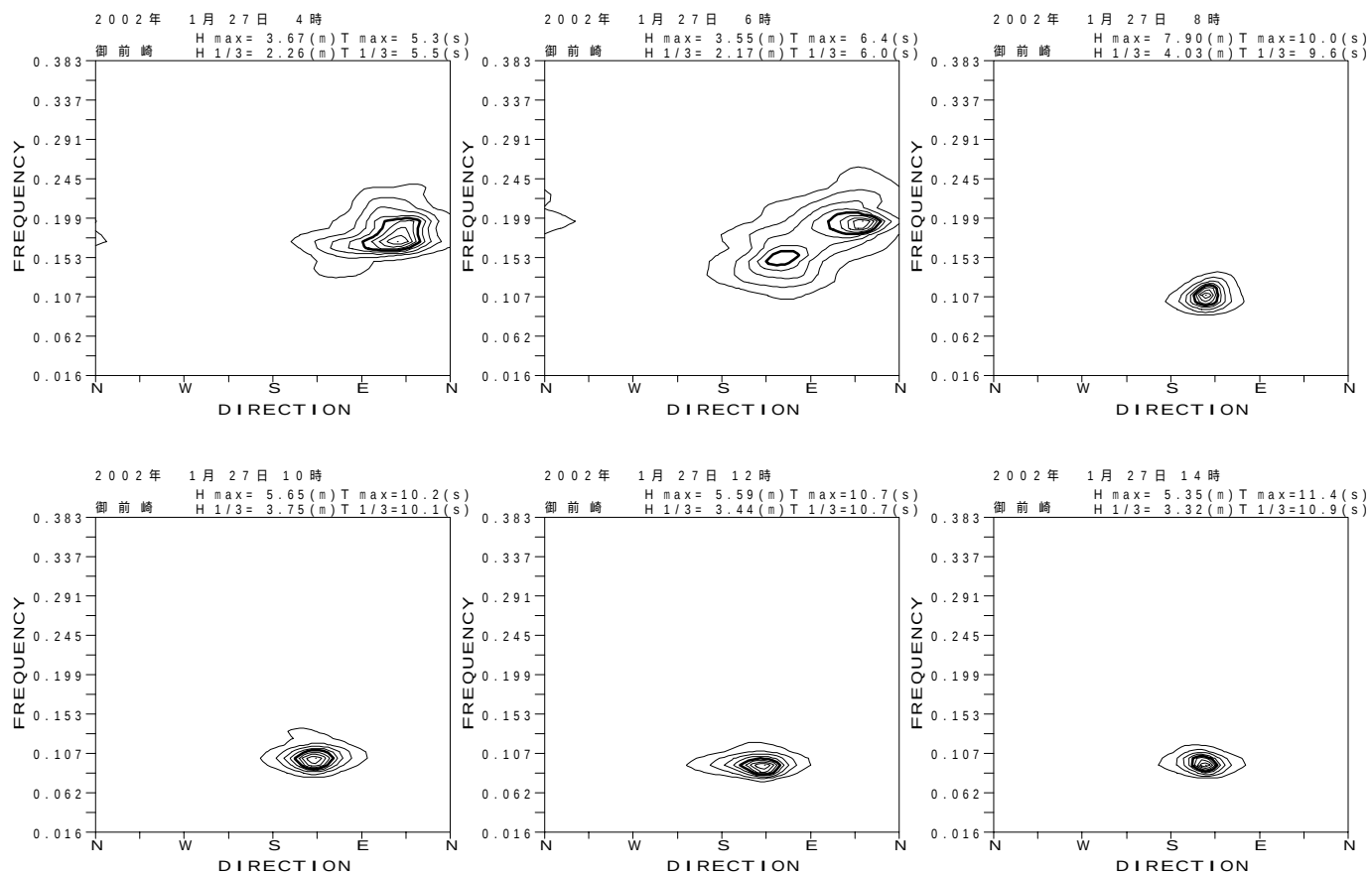
付図 - B.3.40 御前崎 代表的な高波期間中の方向スペクトル
