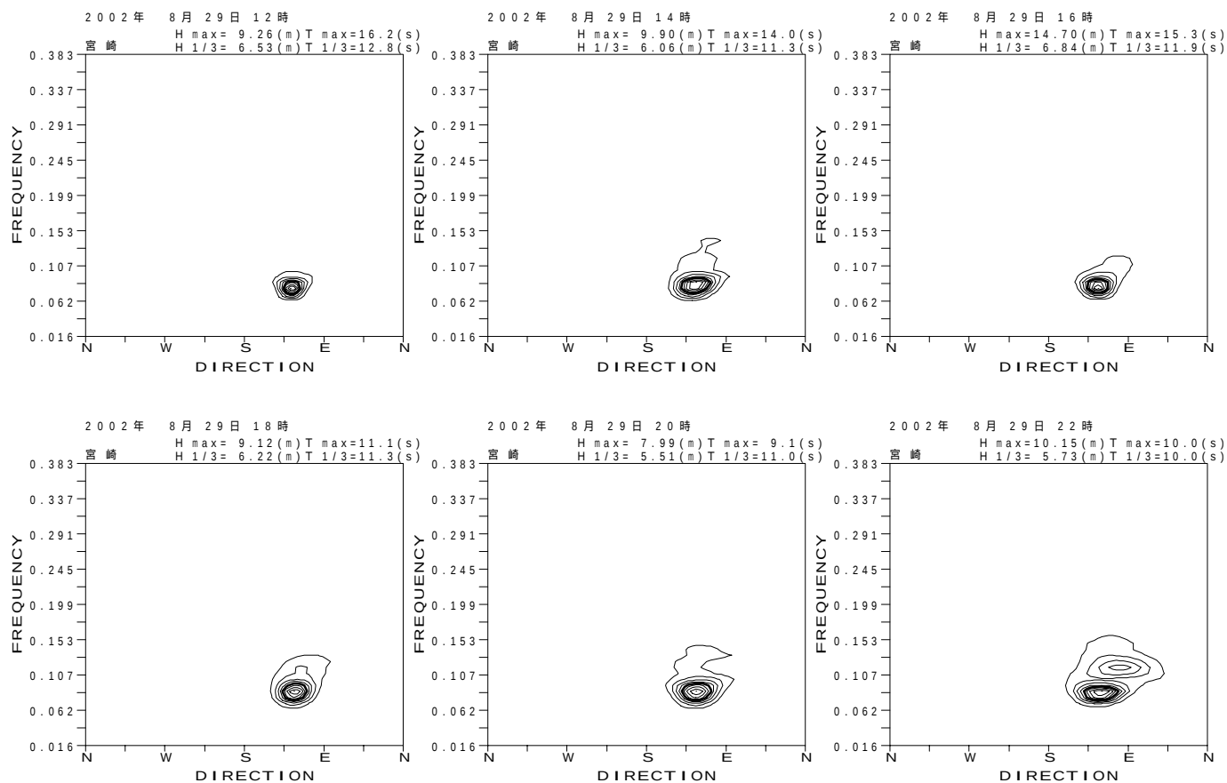
付図 - B.3.50 宮崎 代表的な高波期間中の方向スペクトル
