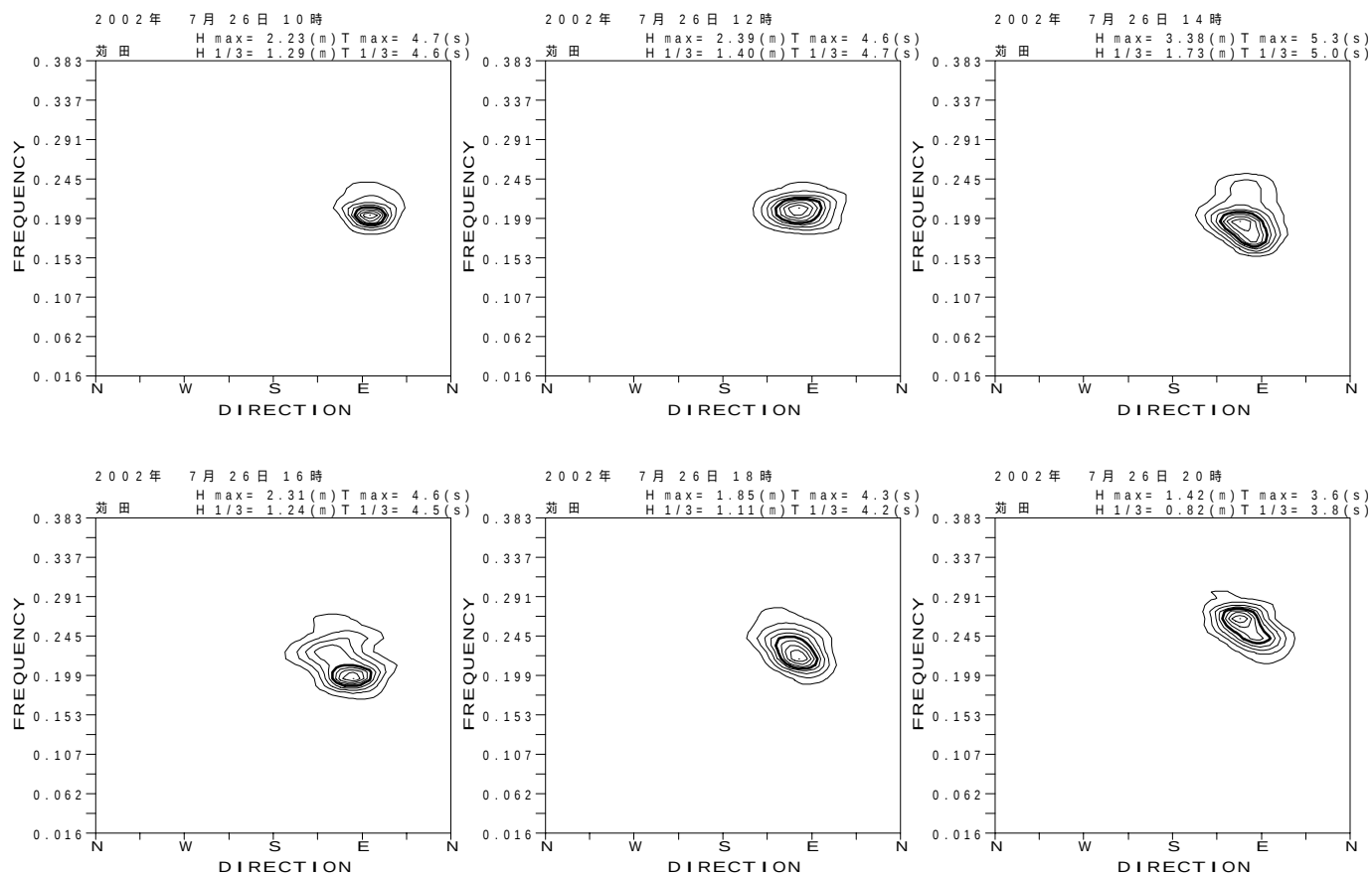
付図 - B.3.48 菊田 代表的な高波期間中の方向スペクトル
