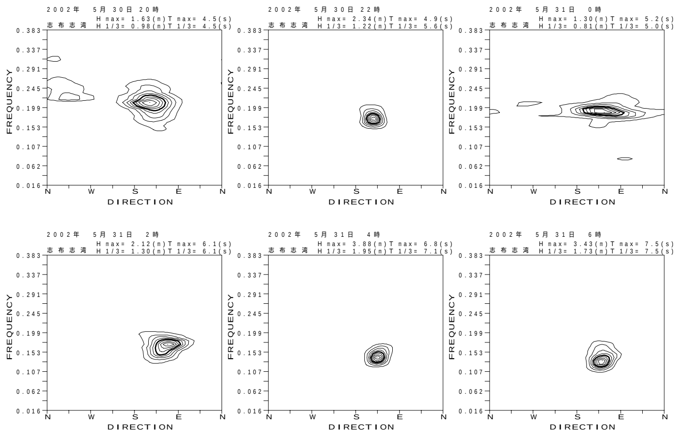
付図 - B.3.51 志布志湾 代表的な高波期間中の方向スペクトル
