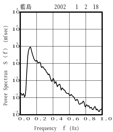
付図-B.3.17 藍島 代表的な高波期間中のスペクトル
