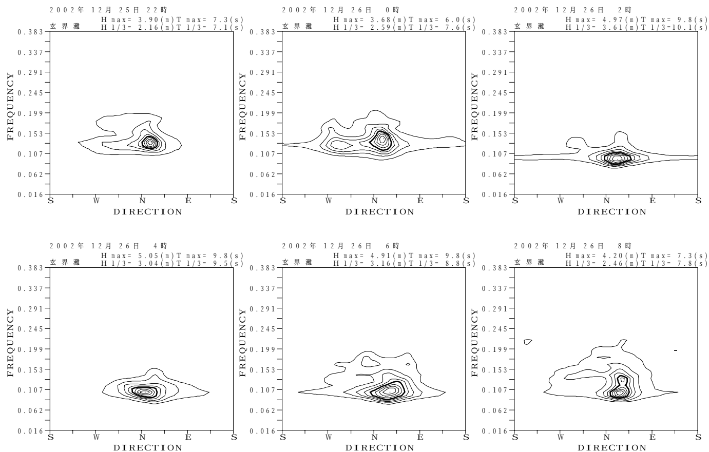
付図-B.3.18 玄界灘 代表的な高波期間中の方向スペクトル
