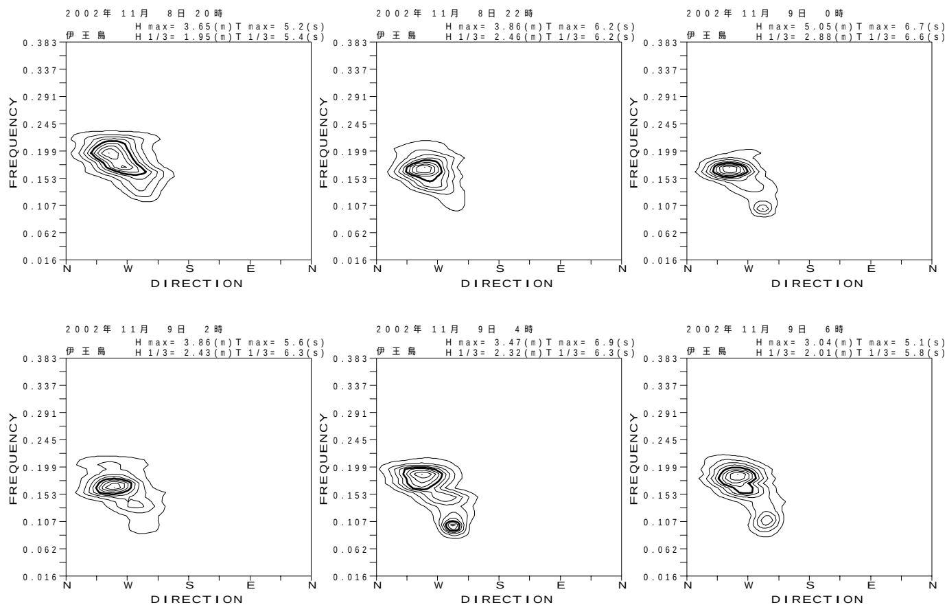
付図 - B.3.19 伊王島 代表的な高波期間中の方向スペクトル
