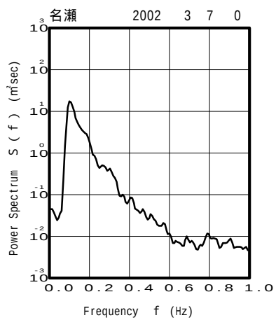
付図 - B.3.20 名瀬 代表的な高波期間中のスペクトル
