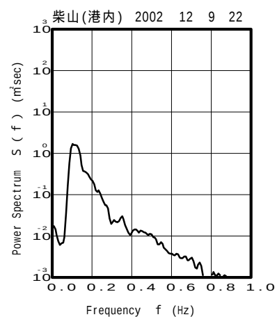
付図 - B.3.13 柴山(港内) 代表的な高波期間中のスペクトル
