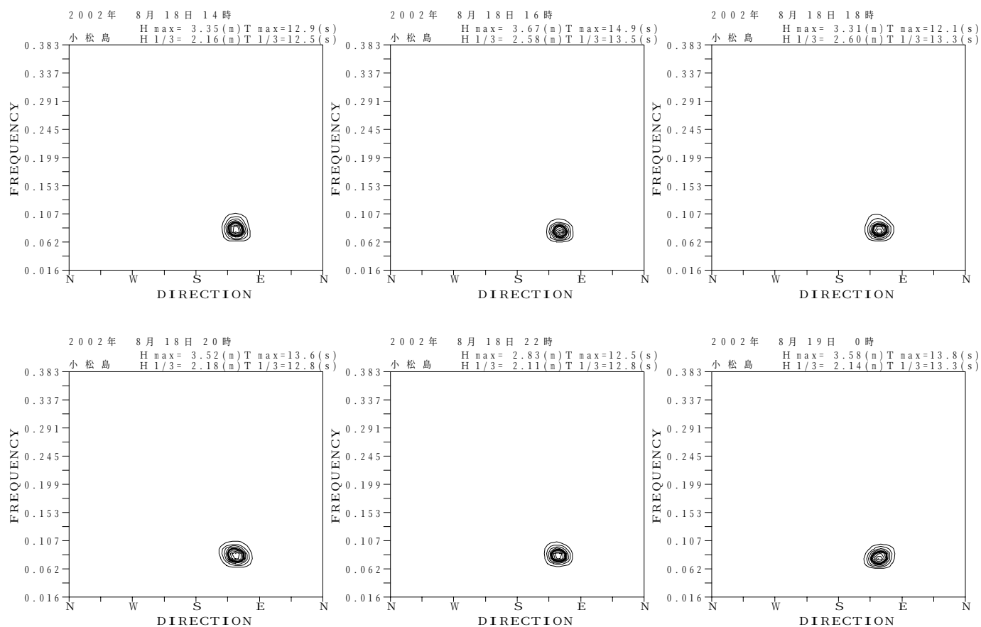
付図－B.3.44 小松島 代表的な高波期間中の方向スペクトル
