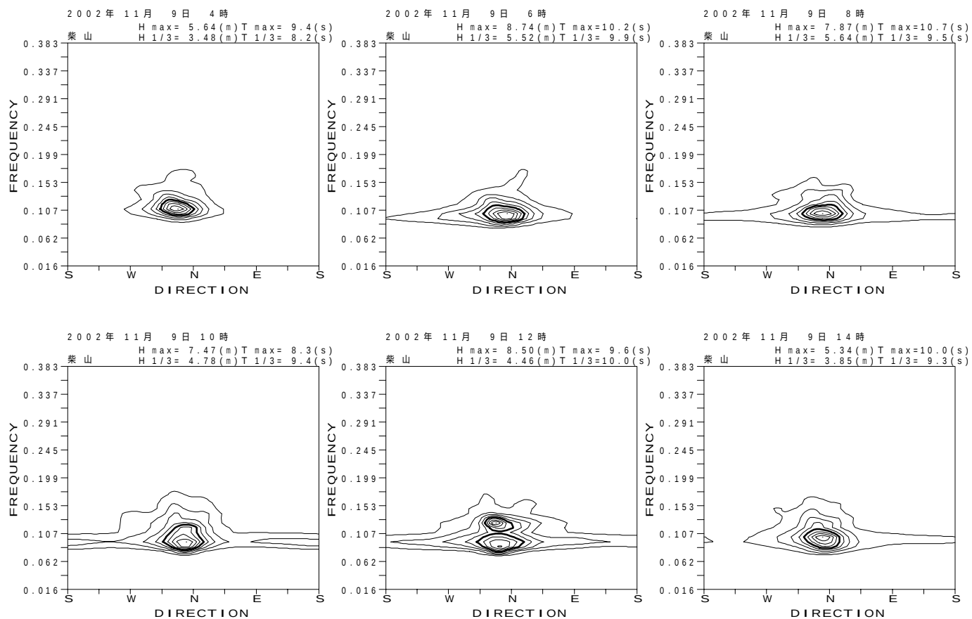
付図 - B.3.12 柴山 代表的な高波期間中の方向スペクトル
