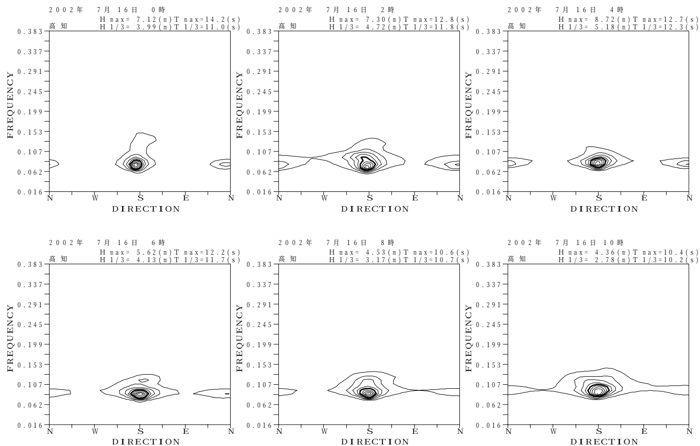
付図－B.3.46 高知 代表的な高波期間中の方向スペクトル
