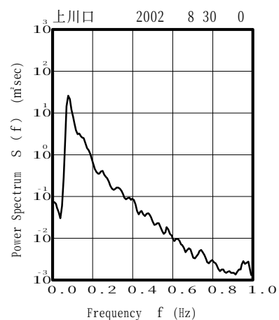
付図-B.3.47 上川口 代表的な高波期間中のスペクトル
