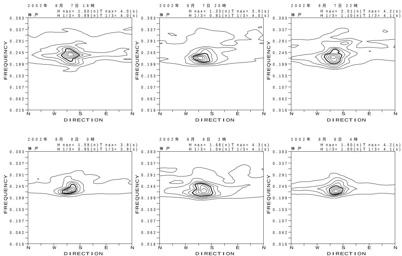
付図 - B.3.43 神戸 代表的な高波期間中の方向スペクトル
