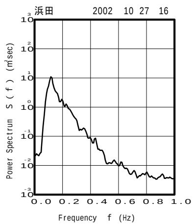
付図 - B.3.16 浜田 代表的な高波期間中のスペクトル
