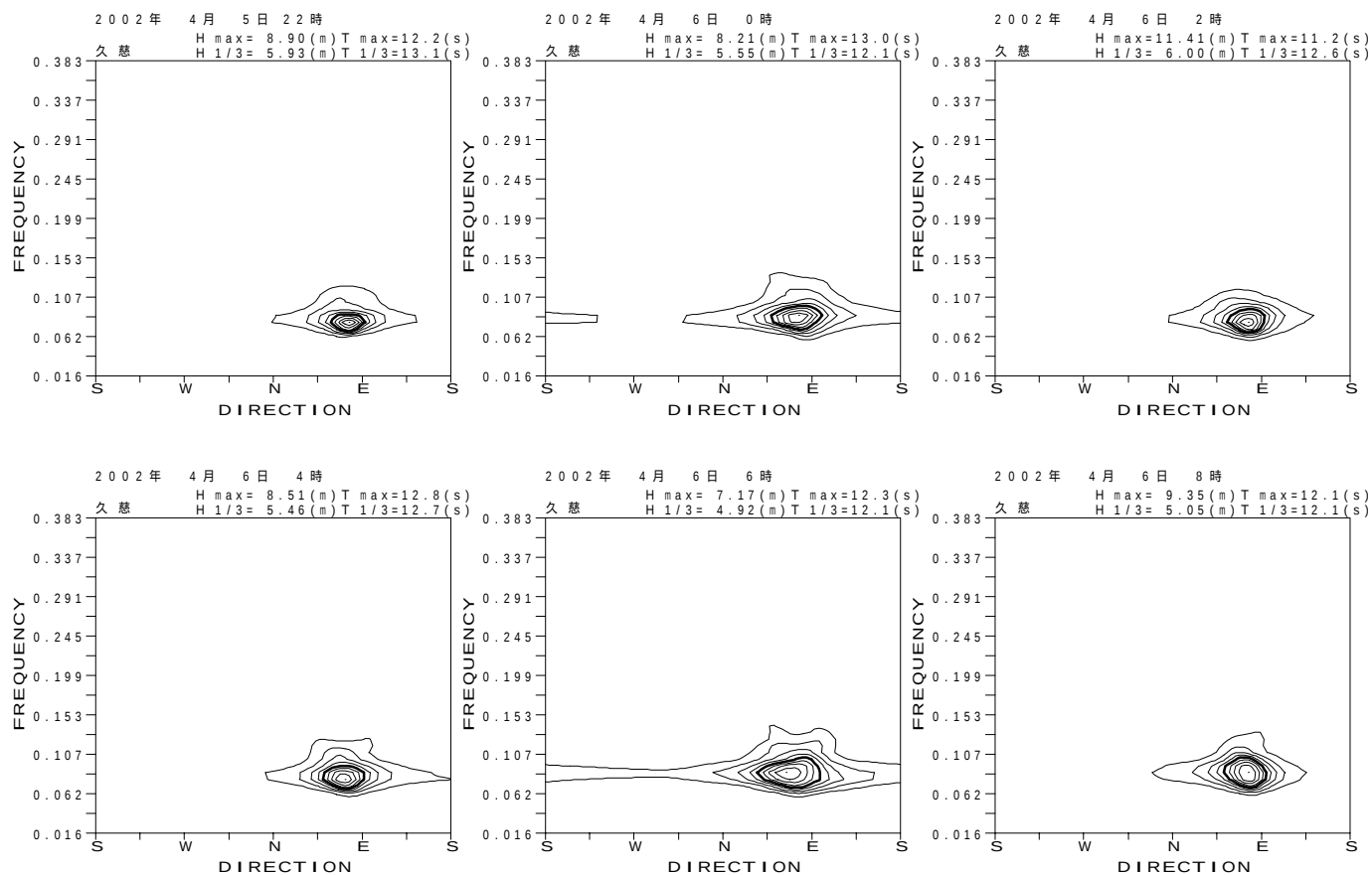
付図 - B.3.27 久慈 代表的な高波期間中の方向スペクトル
