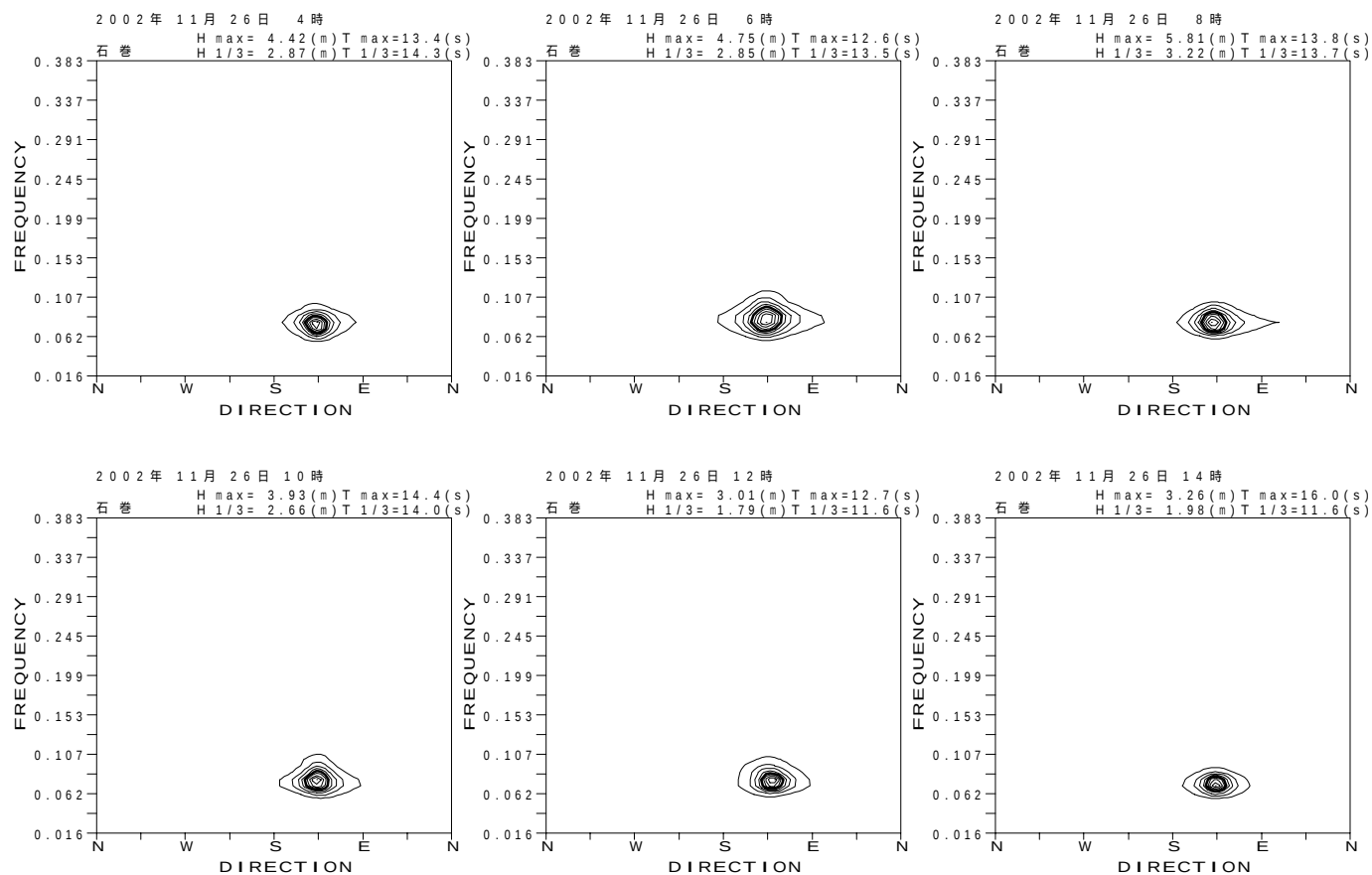
付図 - B.3.29 石巻 代表的な高波期間中の方向スペクトル
