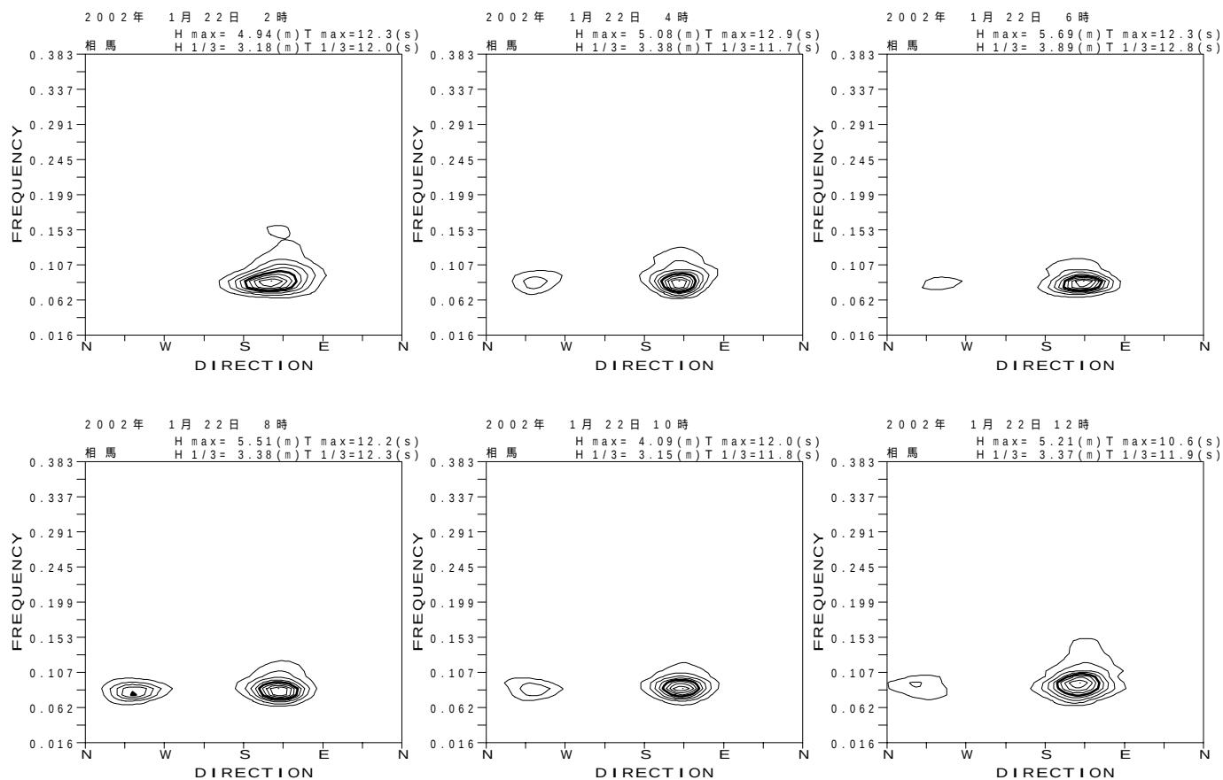
付図 - B.3.31 相馬 代表的な高波期間中の方向スペクトル
